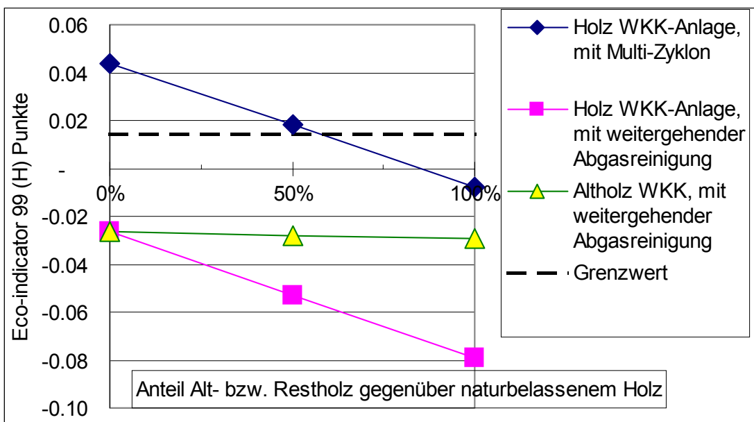
Fig. 18 Einfluss der Brennstoffzusammensetzung auf das Ergebnis für die drei Standardanlagen. Gezeigt wird die Umweltbelastung in Eco-indicator 99 (H) Punkten pro kWh Strom.
