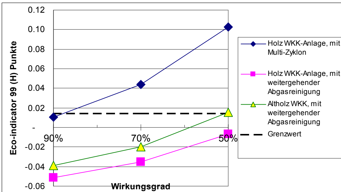
Fig. 19 Einfluss des Gesamtwirkungsgrades auf das Gesamtergebnis für die drei Standardanlagen. Eco-indicator 99 (H) Punkte pro kWh Strom.
