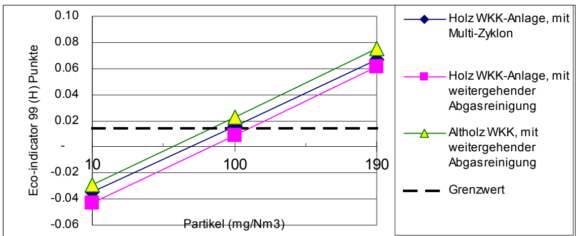
Fig. 16 Einfluss der Partikelemissionen auf das Ergebnis für die drei Standardanlagen. Eco-indicator 99 (H) Punkte pro kWh Strom für die Standardanlagen.
