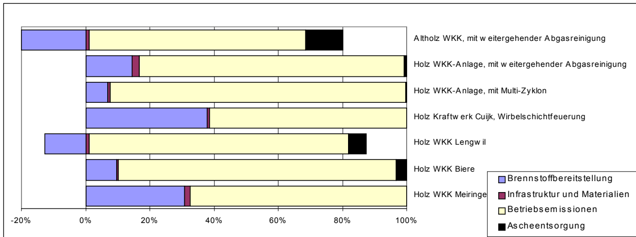
Fig. 12 Dominanzanalyse für die mit dem Eco-indicator 99 (H) bewerteten Umweltbelastungen bezogen auf den Betrieb der vier untersuchten Anlagen und für die drei Standardanlagen.
