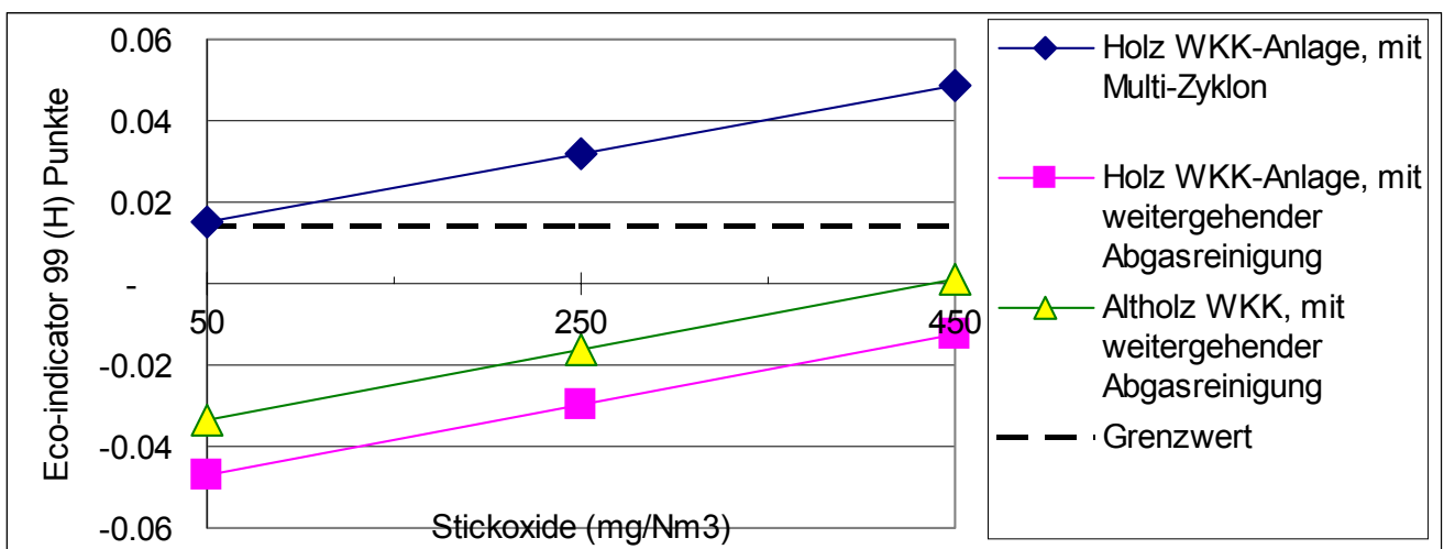
Fig. 17 Einfluss der NO x Emissionen auf das Ergebnis für die drei Standardanlagen. Eco-indicator 99 (H) Punkte pro kWh Strom für die Standardanlagen.
