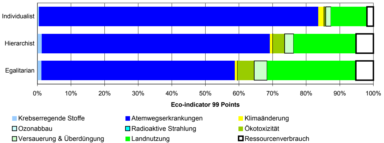
Fig. 13 Anteil der neun Schadenskategorien bei der Bewertung der Umweltbelastungen mit dem Eco-indicator 99 für den Betrieb einer Holz WKK-Anlage mit Multi-Zyklon.
