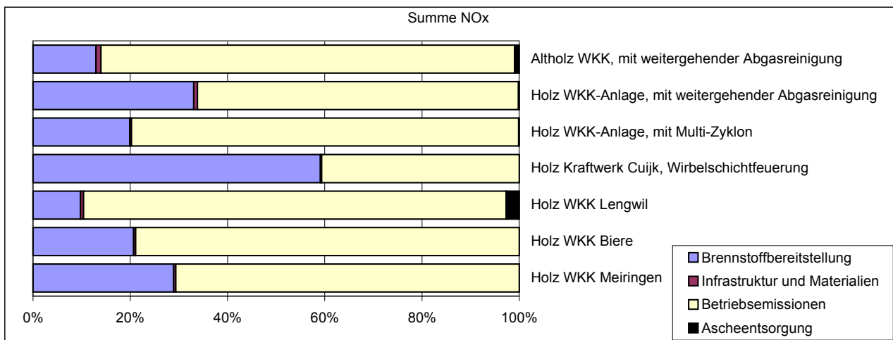
Fig. 10 Dominanzanalyse für die Emission von NO x beim Betrieb der vier untersuchten Anlagen und für die drei Standardanlagen.
